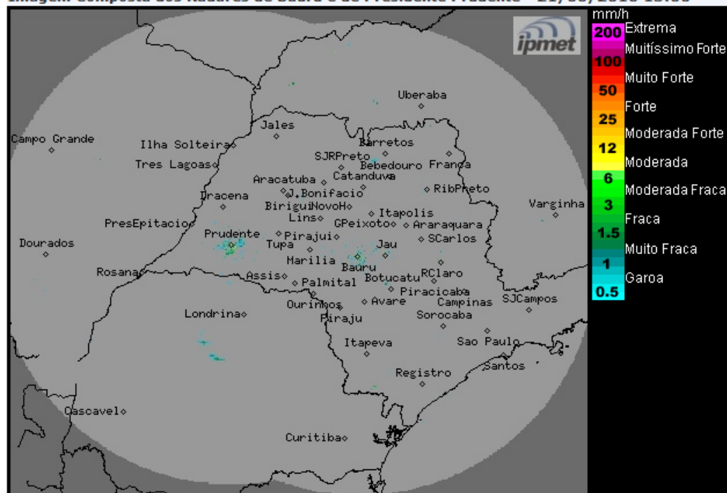
Imagem Composta dos Radares de Bauru e de Presidente Prudente - 21/08/2018 13:00
