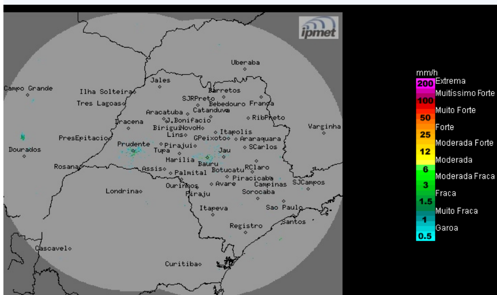
Imagem Composta dos Radares de Bauru e de Presidente Prudente - 12/11/18 14:00
