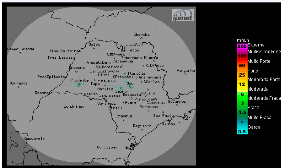
Imagem Composta dos Radares de Bauru e de Presidente Prudente - 18/06/2019 08:00
