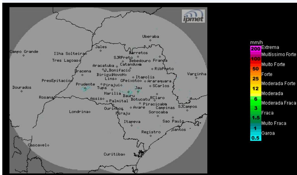
Imagem Composta dos Radares de Bauru e de Presidente Prudente - 25/06/2019 08:00
