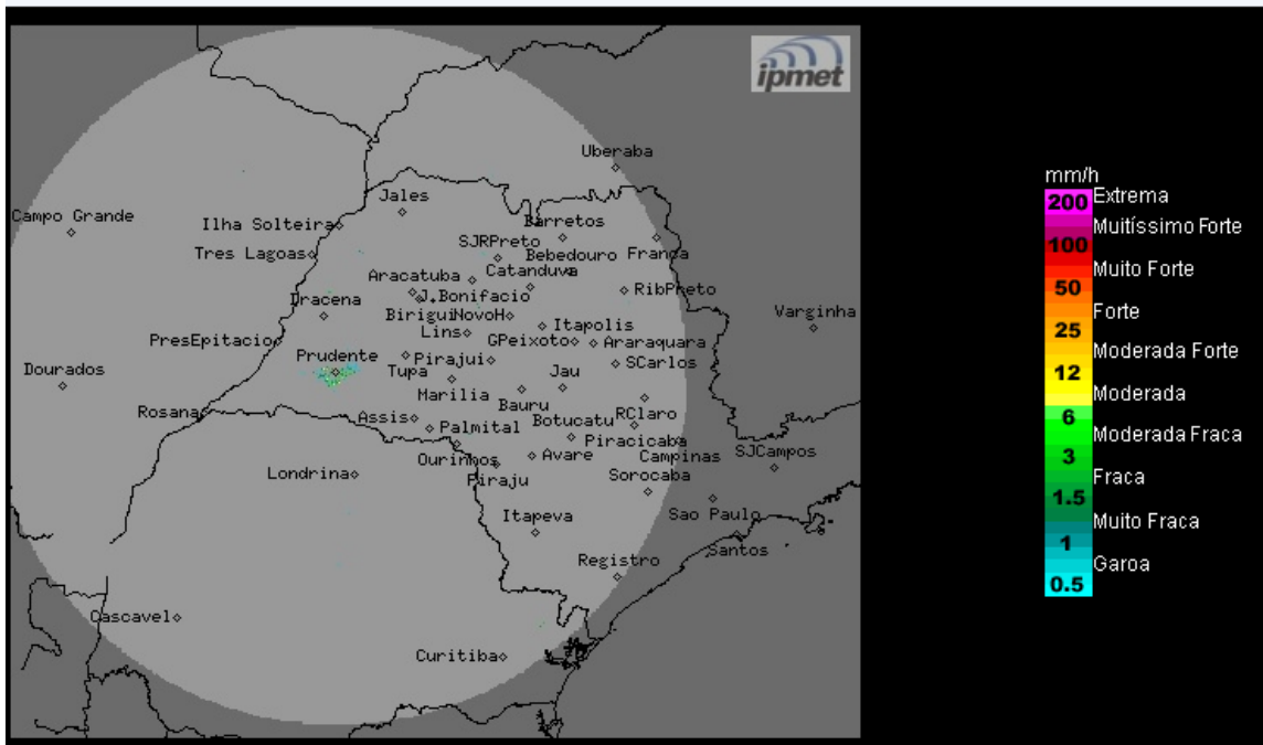
Imagem Composta dos Radares de Bauru e de Presidente Prudente - 17/02/2020 08:45
