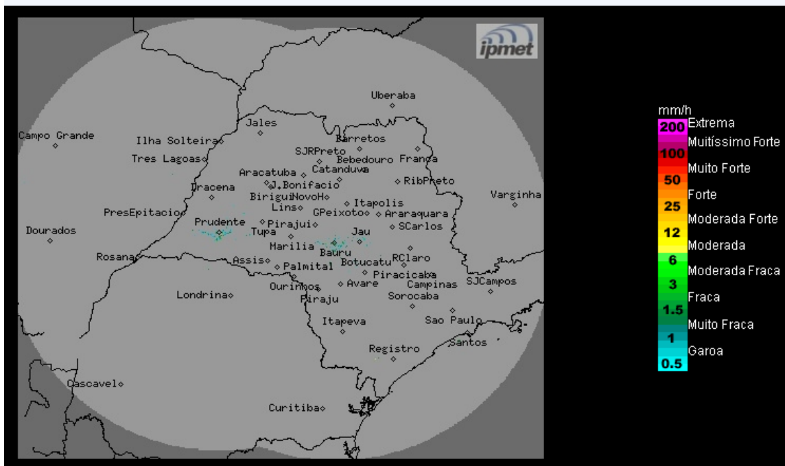
Imagem Composta dos Radares de Bauru e de Presidente Prudente - 24/06/2020 08:00
