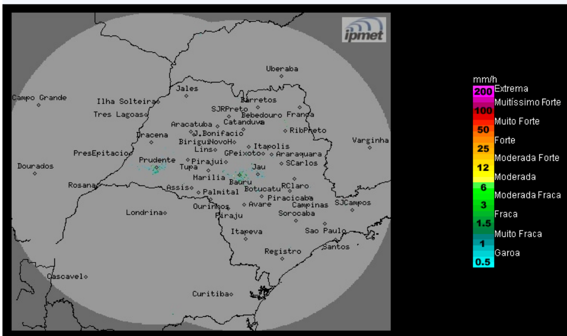
Imagem Composta dos Radares de Bauru e de Presidente Prudente - 02/07/2020 08:00
