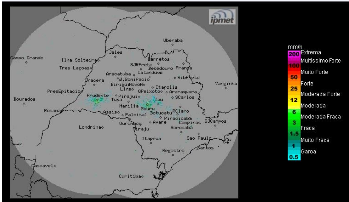
Imagem Composta dos Radares de Bauru e de Presidente Prudente - 04/11/2020 09:00
