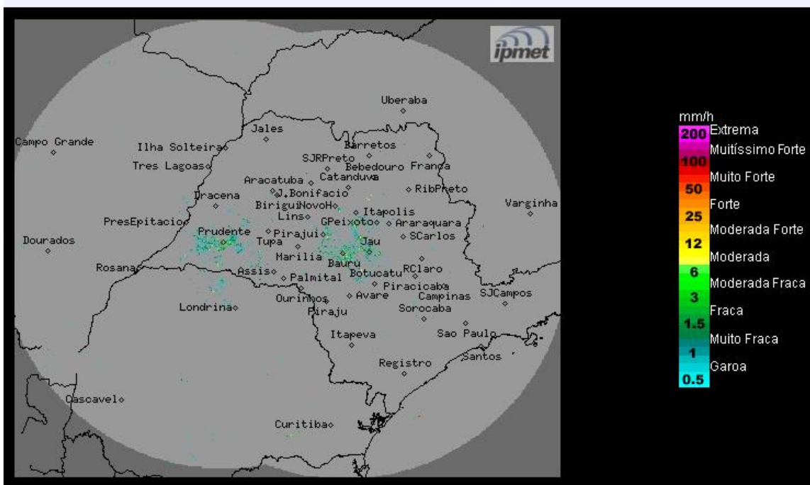
Imagem Composta dos Radares de Bauru e de Presidente Prudente - 21/09/2021 08:00
