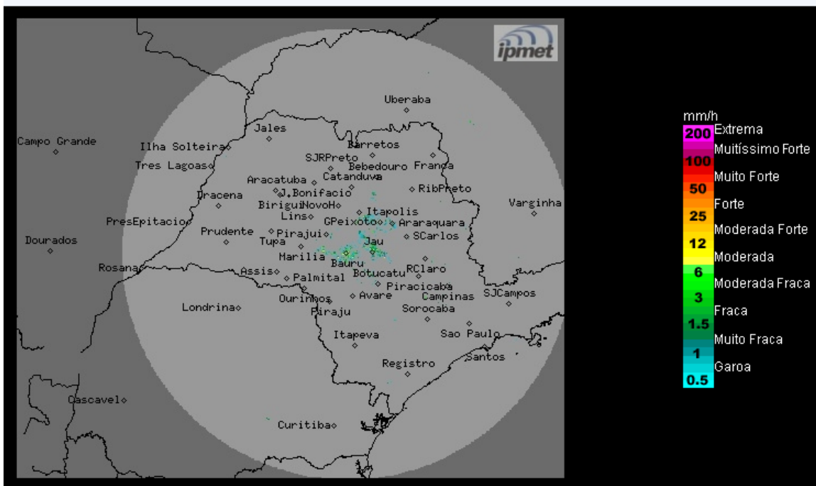
Imagem Composta dos Radares de Bauru e de Presidente Prudente - 23/05/2022 09:00
